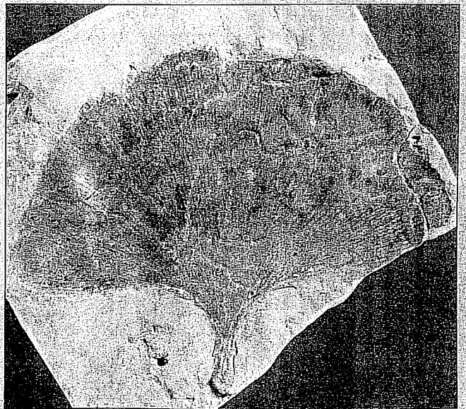
Versteinertes Ginkgoblatt von einem Fundort nahe Freising
